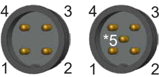
针脚连接示意图（前视图）
